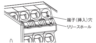
形E5DC-B
