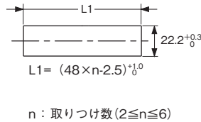
横密着取り付け時
