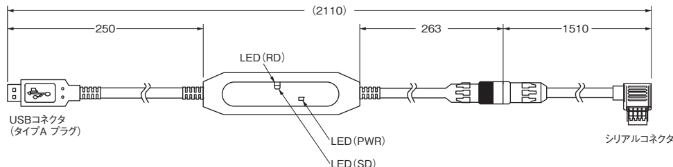
形E53-COV23(3ヶ詰め)
