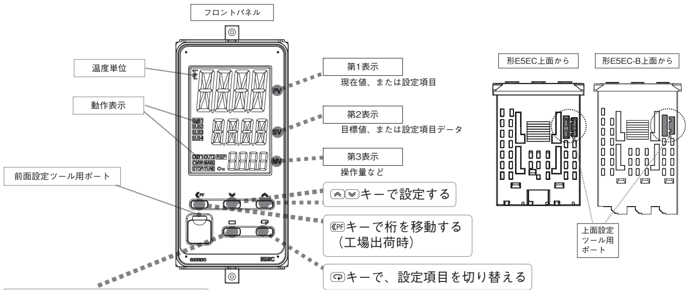
形E5EC/形E5EC-B
