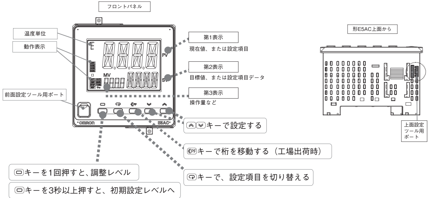
形E5AC
