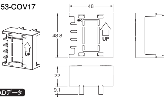
形E53-COV17
