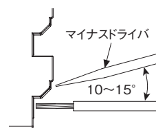
形E5DC-B
