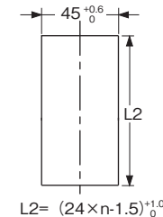
縦密着取り付け時
