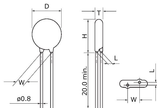
(ERZV10D182CS)
