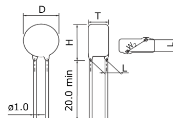
(ERZV20D182)
