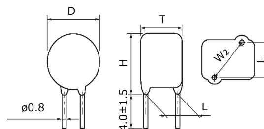
(ERZV10D182CS)
