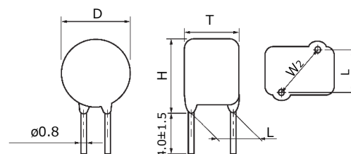
(ERZV14D182CS)
