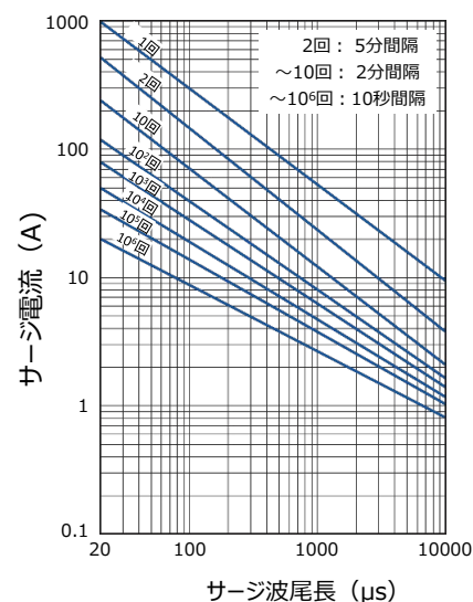
ERZV10D180 ~ ERZV10D680
