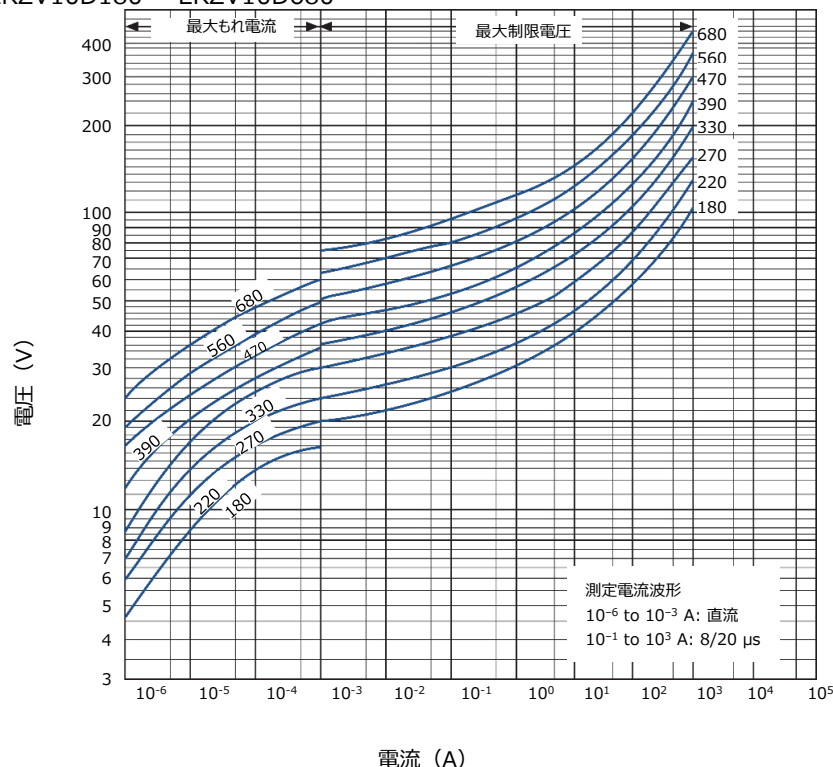
ERZV10D180 ~ ERZV10D680
