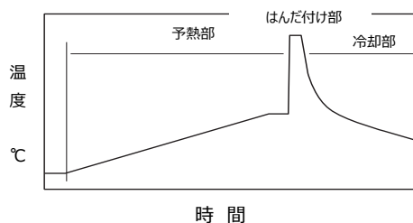
フローソルダリング（はんだ浴浸漬法）
