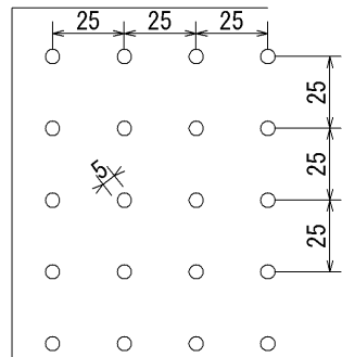
NF-M, NF-817S パネル(1.0t 鉄板製) の穴配置図
