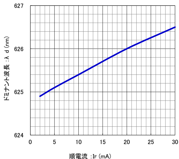
順電流 vs. ドミナント波長
