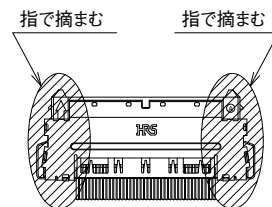
③ 指でつまんで組み込む
