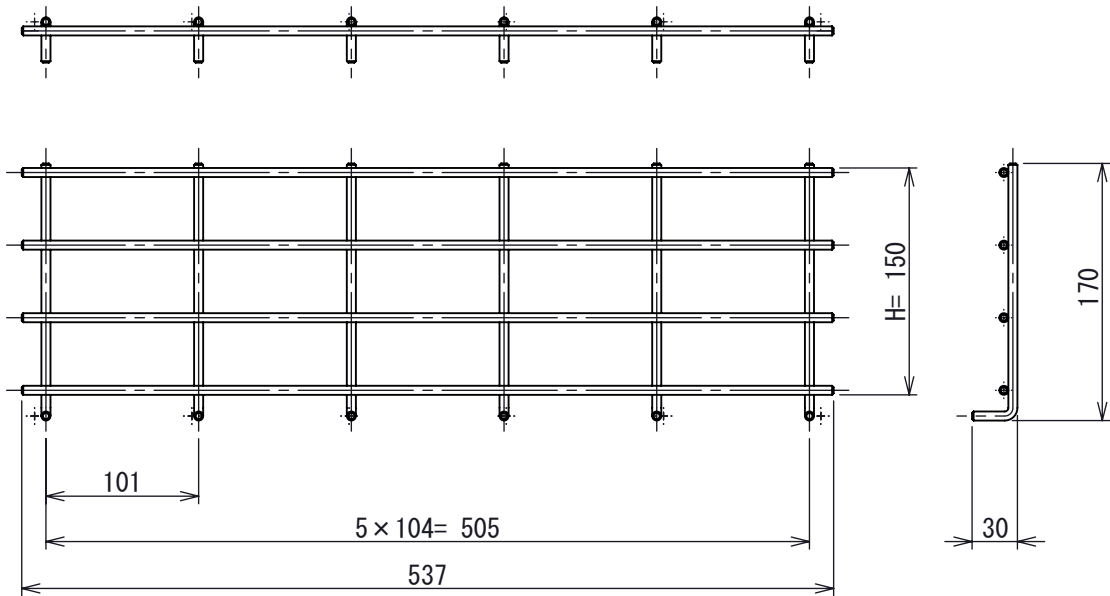
部品② ガードフェンス側面H150用 詳細
