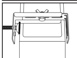
① 塀のサイズや状態を確認し、アジャスターの位置を決め（図Aを参照）各部品を仮止めしてください。
