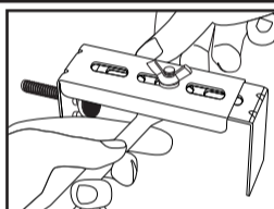
② 上部のネジを確実に固定してください。
