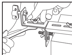
⑥ 金具が塀にしっかり固定出来ているか確認し、ミラーを取り付けてください。（確実に固定してください）
