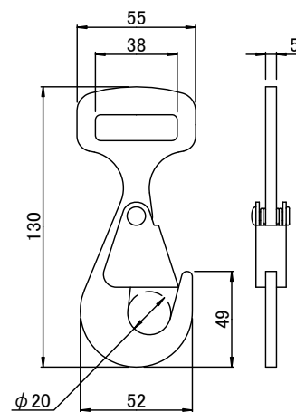
スナップフック
