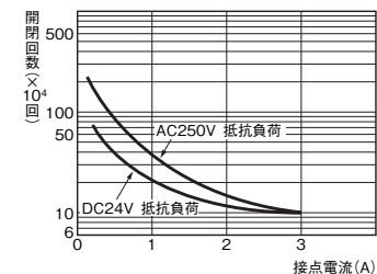
形H3YN-4-Z/-41-Z
