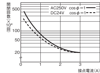
形H3YN-4/-41
