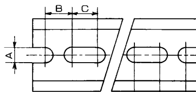
寸法図
