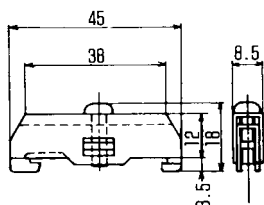
寸法図
