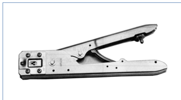
手動圧着工具 HIF3-T2226HC
