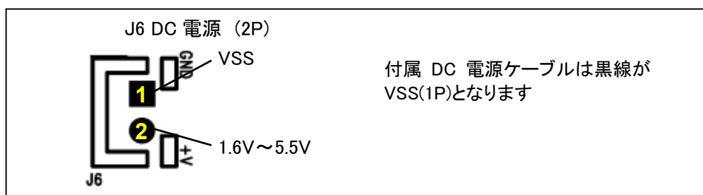
図 2-2 DC 電源図
