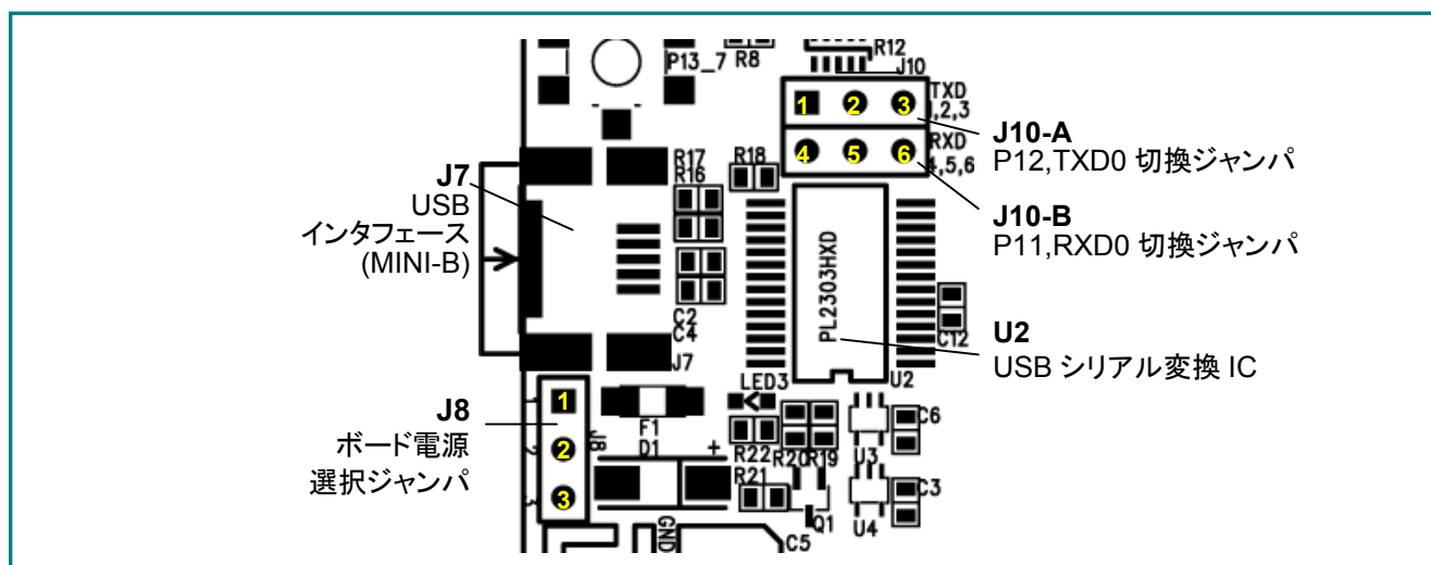
図 1-2 ボード配置補足図
