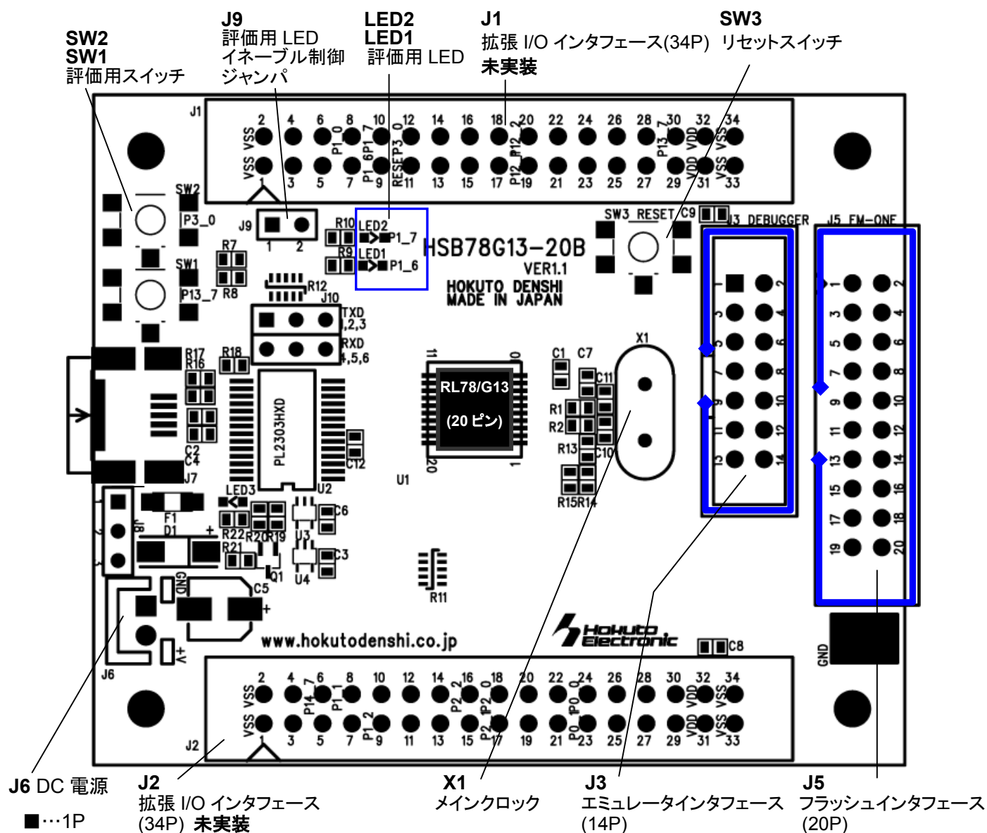
図 1-1 ボード配置図
