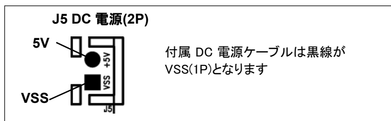
図 2-2 DC 電源図
