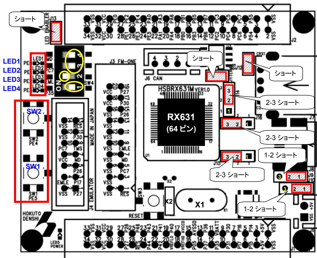
図 5-1 初期設定図
