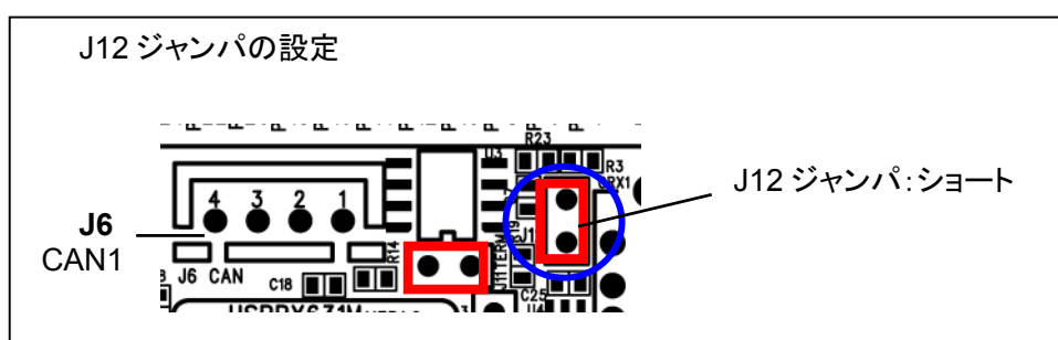
図 2-8 CAN1 受信信号接続ジャンパ設定図(J12)
