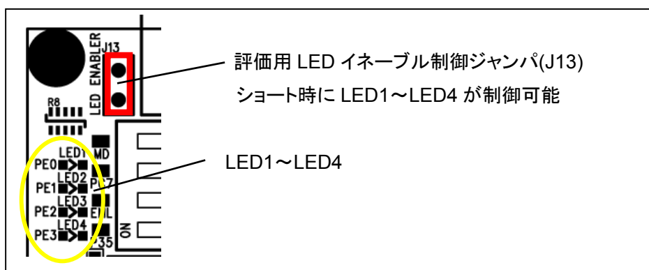
図 2-10 評価用 LED イネーブル制御ジャンパ設定図(J13)
