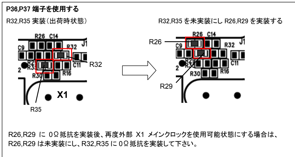
図 2-9 R26,R29,R32,R35 抵抗設定図
