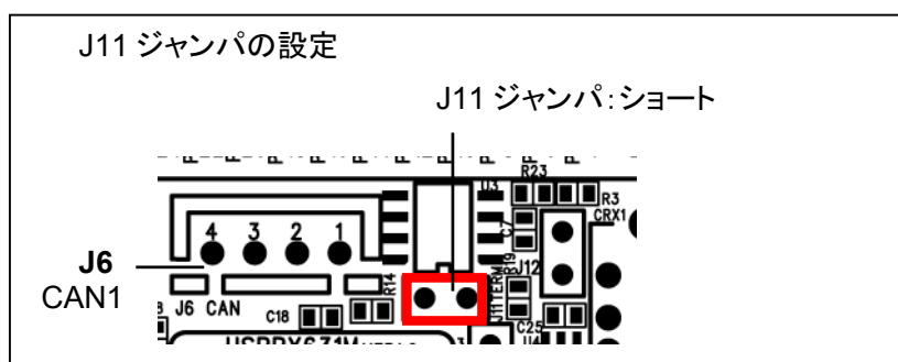
図 2-7 CAN 終端抵抗イネーブル制御ジャンパ設定図(J11)
