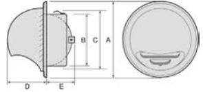
特定防火設備該当品 防火ダンパー付き*2*3
