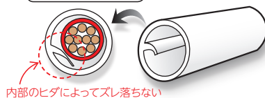
電線挿入時断面図
