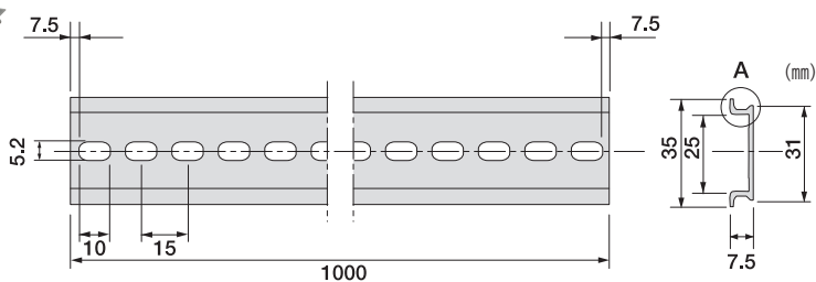
A部詳細
