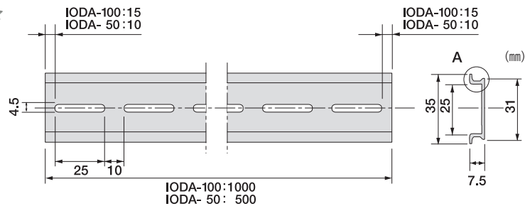
A部詳細
