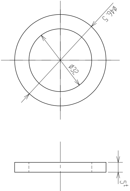
パッキン詳細 ( N R )
