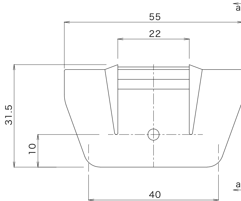
正面図
