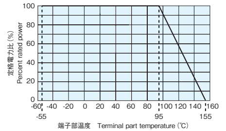
端子部温度 RK73H W3A2
