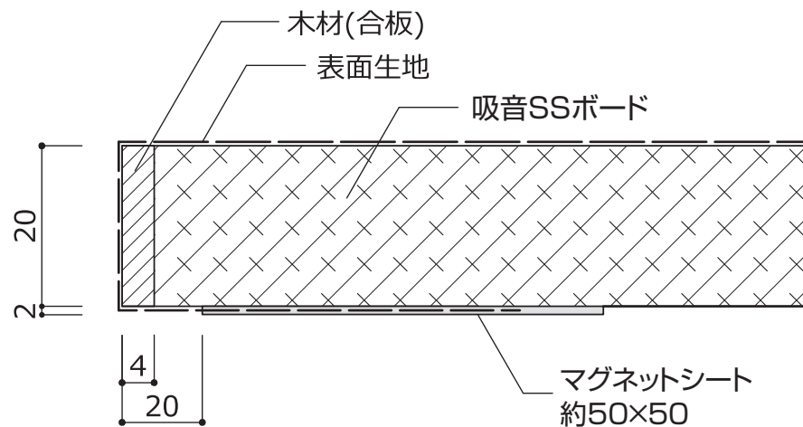
断面詳細図 S=1:1
