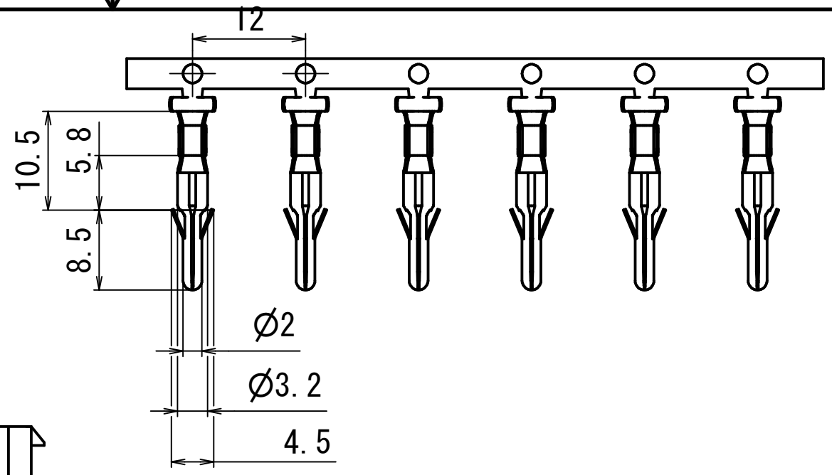
端子 (6 連)
