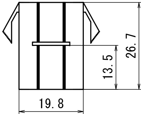
ハウジング
