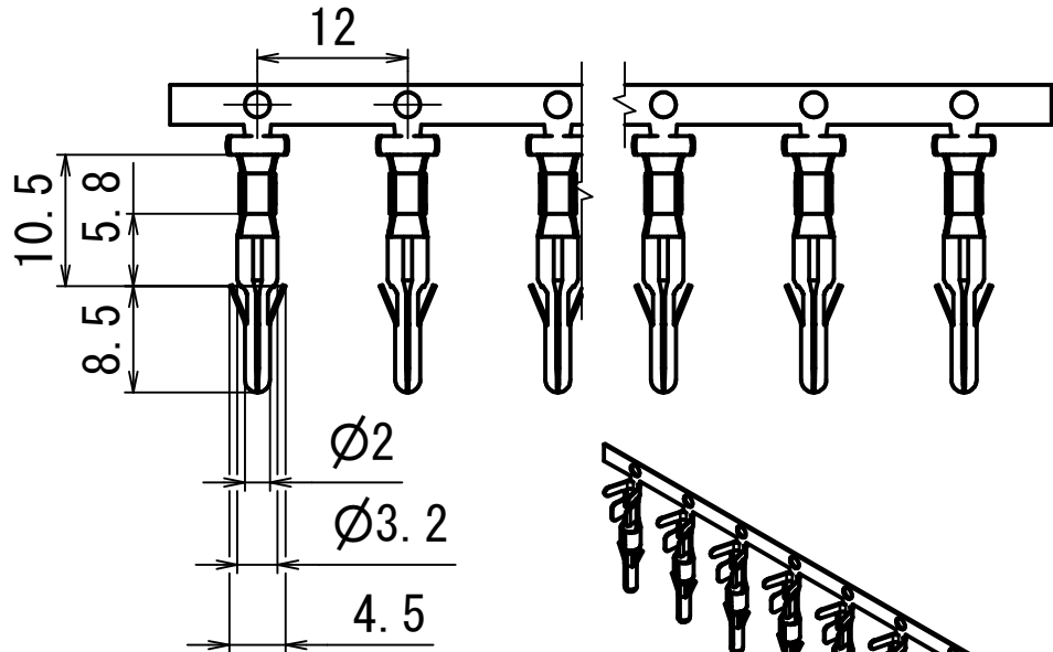
端子 (9連)
