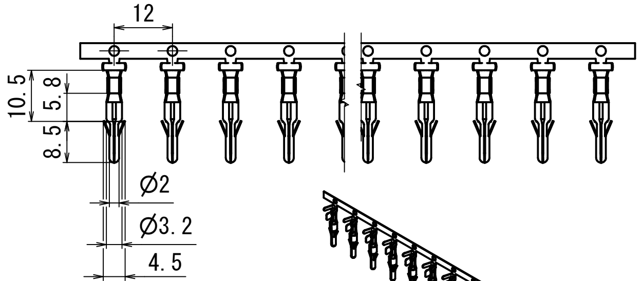
端子 (15連)
