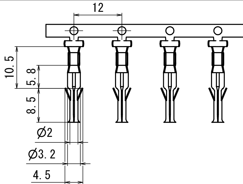
端子 (4連)
