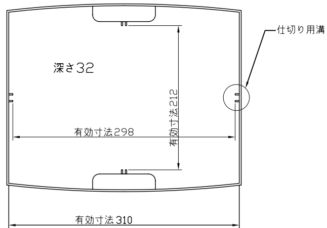
引き出し本体上面図
