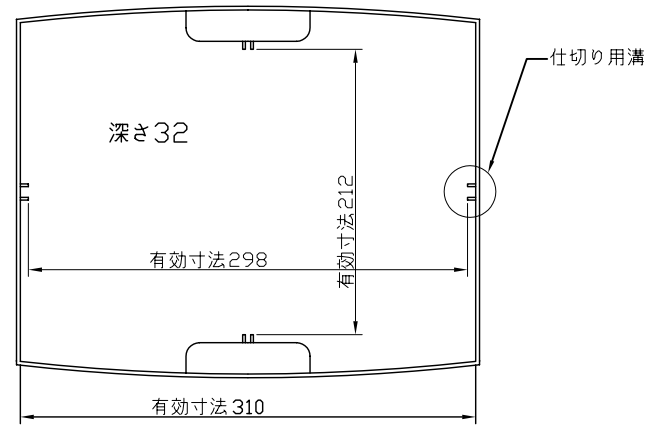
引き出し本体上面図
