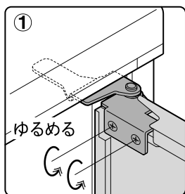
① ヒンジを固定した扉のネジをゆるめる。
