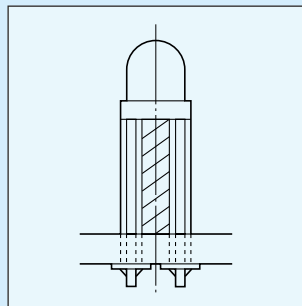
取付例
