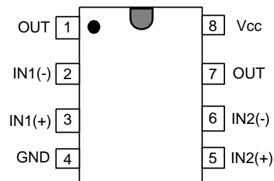
DIP-8
