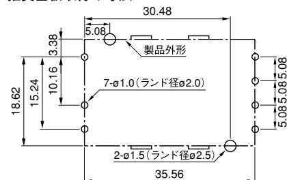
推奨基板取付け寸法
