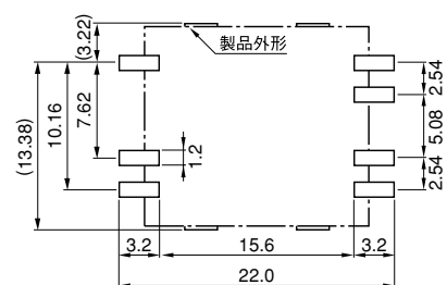
推獎基板取付け寸法
