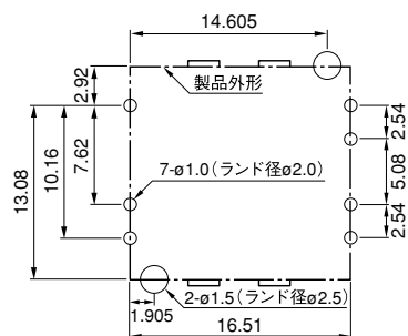
推獎基板取付け寸法
