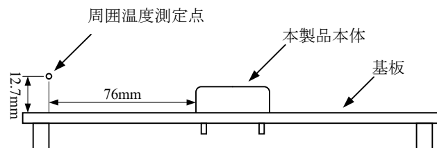
図7-1 周囲温度に対する出力ディレーティングの測定方法(自然空冷の場合)
