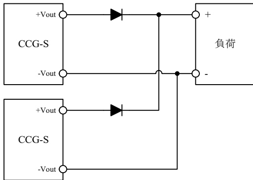
図6-7 冗長運転接続方法 (CCG-S)
