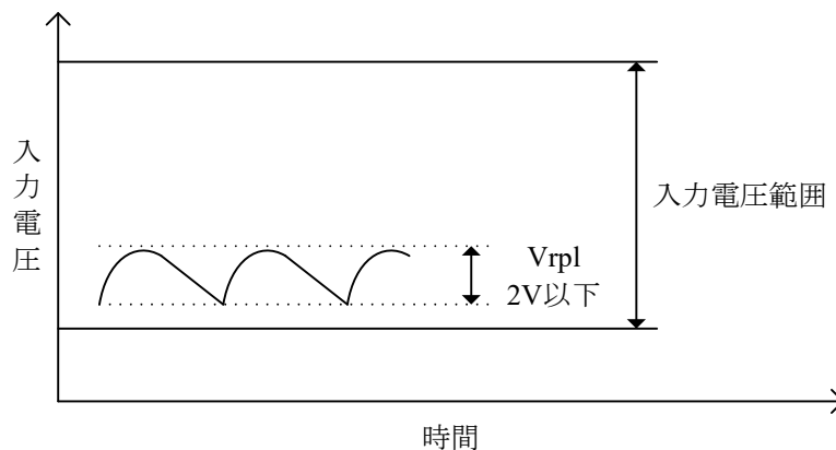
図6-1 入力リップル電圧
