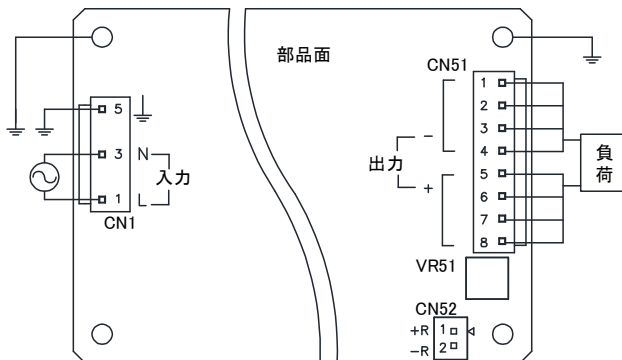
ZWS100BAF
