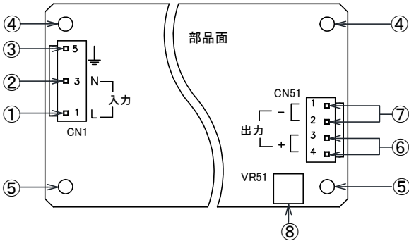
ZWS50BAF
