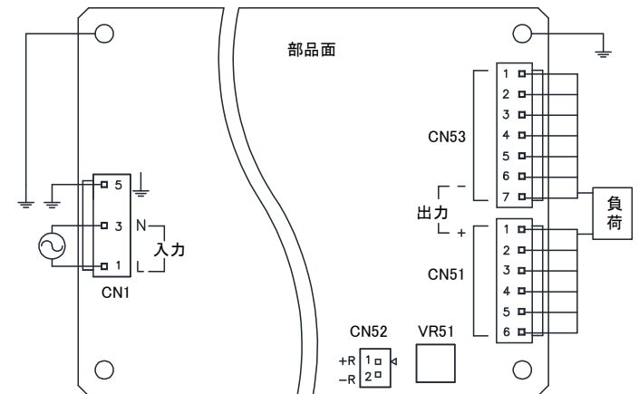
ZWS150BAF
