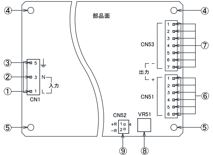
ZWS150BAF
