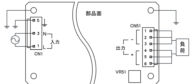
ZWS75BAF
