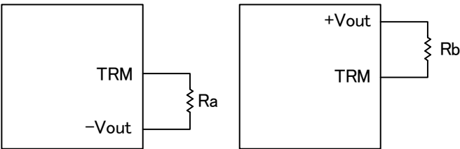
図6 TRM端子抵抗接続方法
