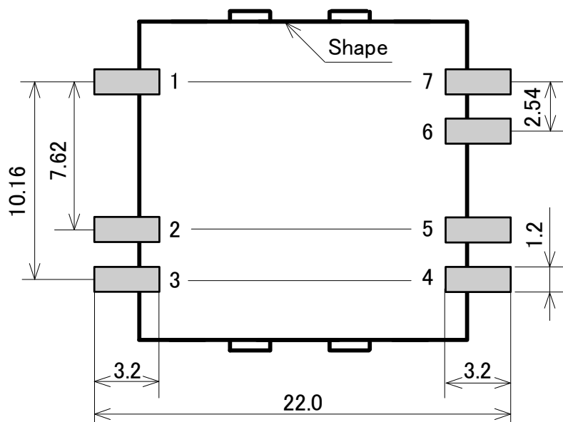
図 13 推奨基板取り付け寸法 (TOP View)
