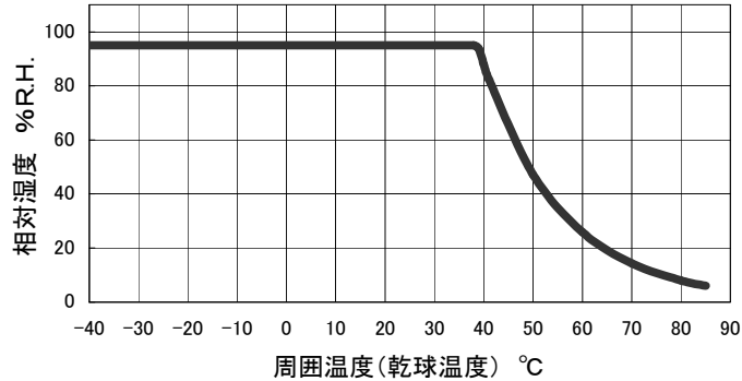
図2 湿度デレーティングカーブ
