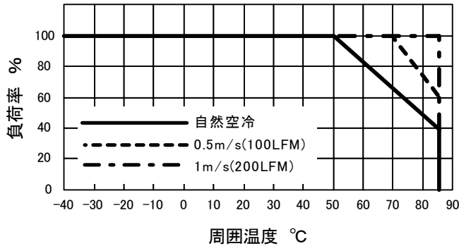
図1 出力デレーティングカーブ
