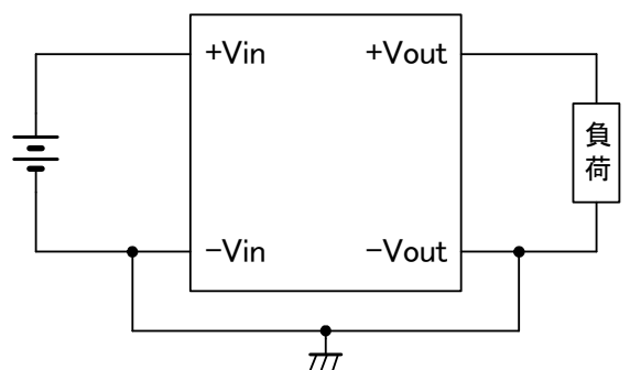
図10 非絶縁で使用する場合の接続
