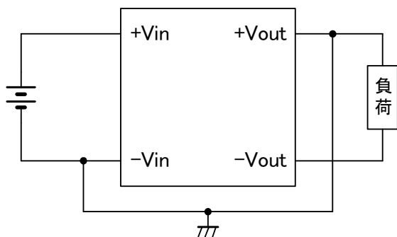
図11 極性反転出力(非絶縁)で使用する場合の接続
