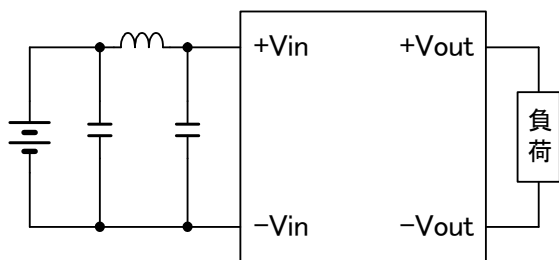
図7 入力リップルノイズを低減する接続
