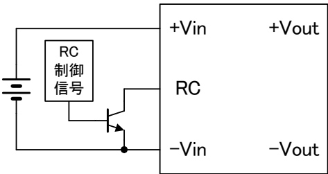
図5 RC端子接続方法
