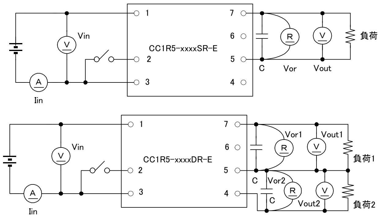
図 3 測定回路図
