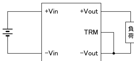
図10 非絶縁で使用する場合の接続
