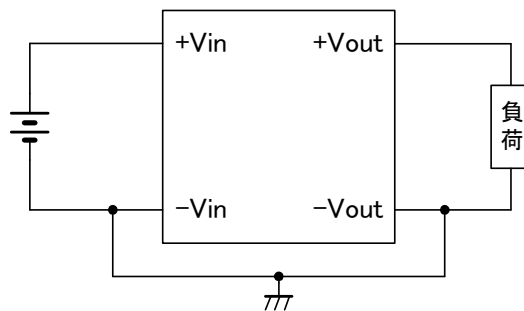
図10 非絶縁で使用する場合の接続
