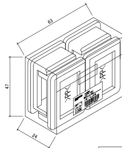
梱包図
