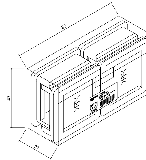
梱包図
