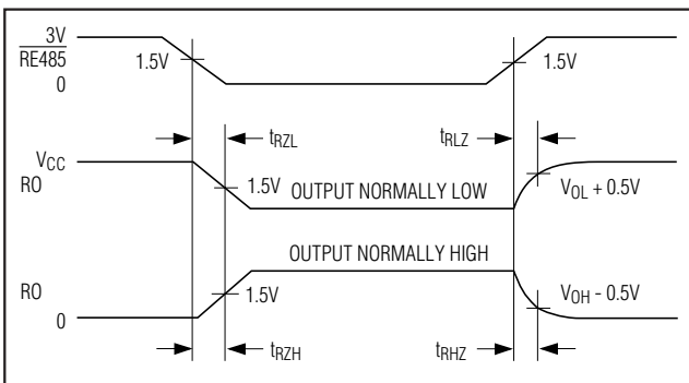
図8. MAX3162 RS-485/422レシーバイネーブル 及びディセーブル時間
