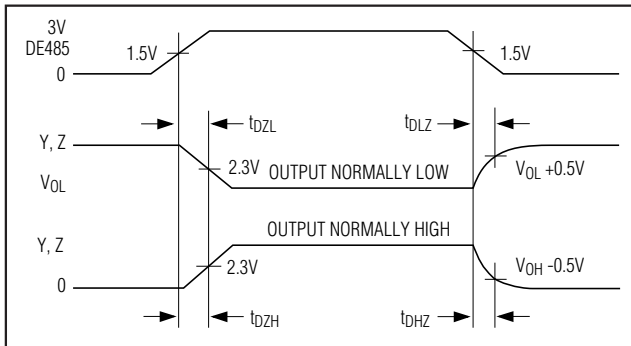
図6. RS485/422ドライバインエーブル及びディセーブル 時間
