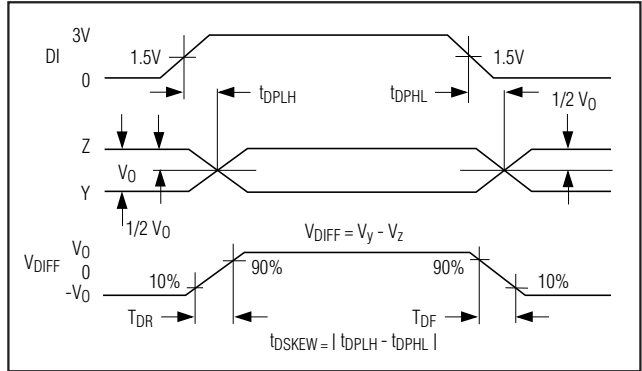
図5. RS-485/422ドライバ伝播遅延
