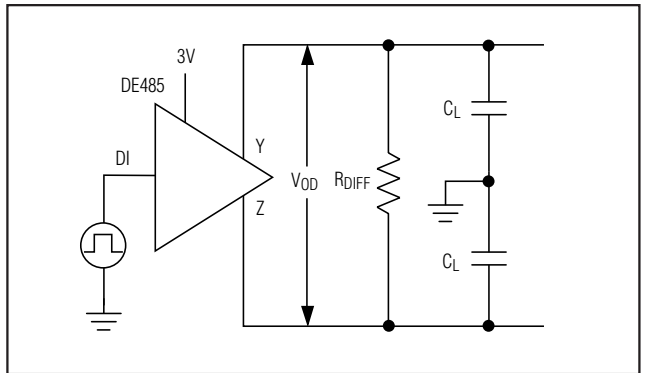
図3. RS-485/422ドライバタイミング試験負荷
