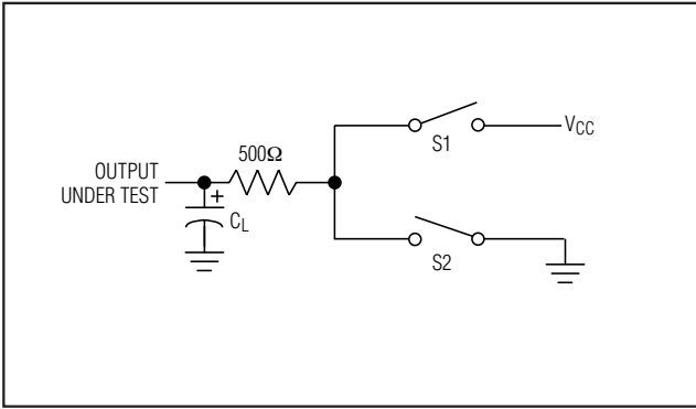
図4. RS-485/422ドライバインエーブル/ディセーブル タイミング試験負荷
