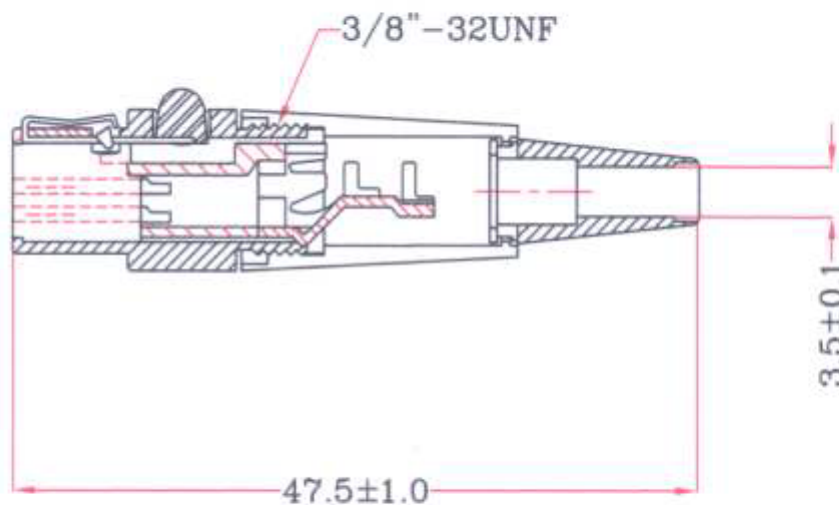
A-A SECTION
