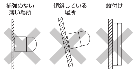
調光器付壁スイッチ(代表例)
