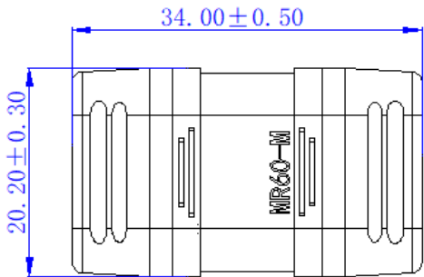
带后盖互配尺寸
