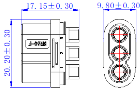
带后盖堆叠尺寸
