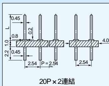
H寸法はMXW-3シリーズとMEW-3-1シリーズ (75ページ参照) を組合せた時のプリント板同志の間隔です。
