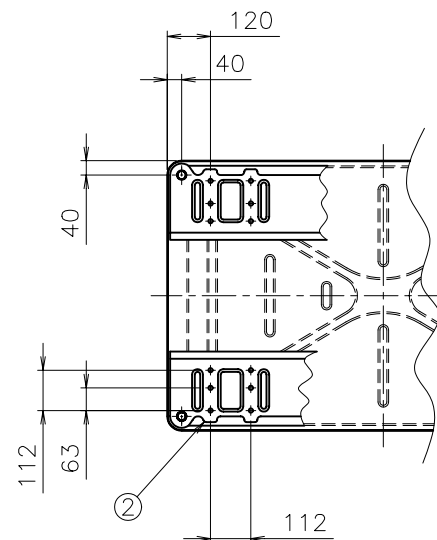
裏面詳細図
