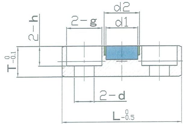
ザグリ穴長円マグネット(サマリウムコバルト磁石)規格表
