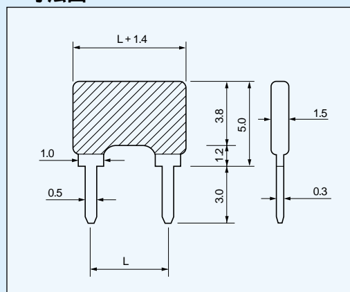
寸法図
