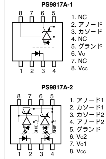
端子接続図 (Top View)
