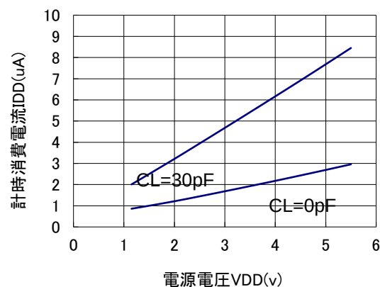
計時消費電流 vs 電源電圧特性(32K クロック出力時) (出力=Open, T_{opt}=25^{\circ}\text{C} )
