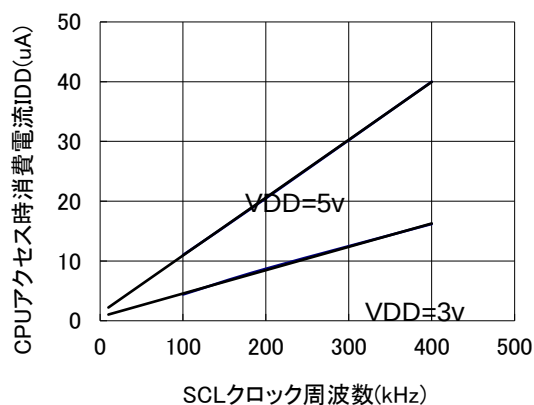
CPU アクセス時消費電流 vs SCL クロック周波数特性 (出力=Open, T_{opt}=25^{\circ}\text{C} , プルアップ電流含まず)
