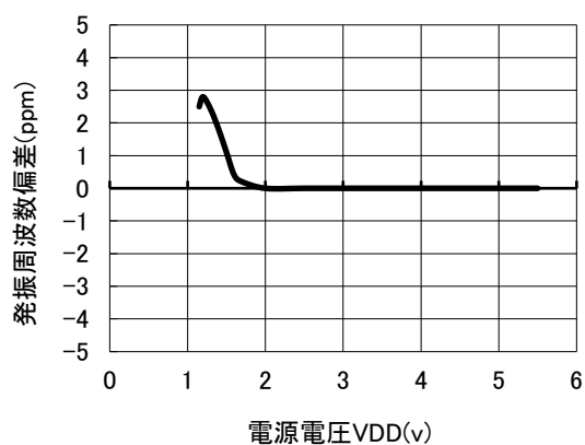
発振周波数偏差 vs 電源電圧特性 ( T_{opt}=25^{\circ}\text{C} , V_{DD}=3\text{V} 基準)
