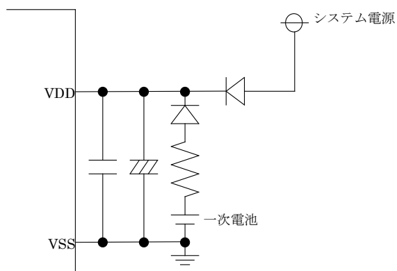
回路例 2
