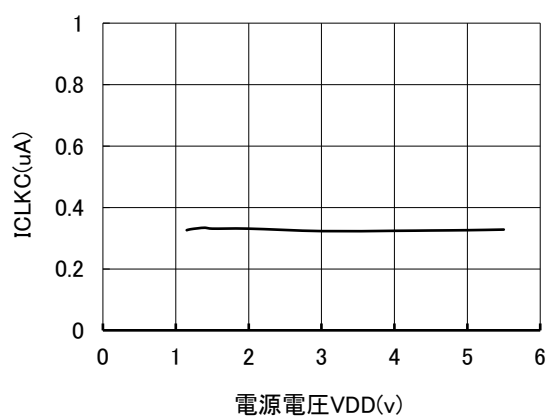
CLKC 端子入力電流 vs 電源電圧特性 ( V_{IN}=V_{DD} , T_{opt}=25^{\circ}\text{C} )
