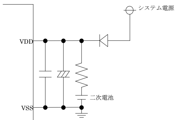
回路例 3
