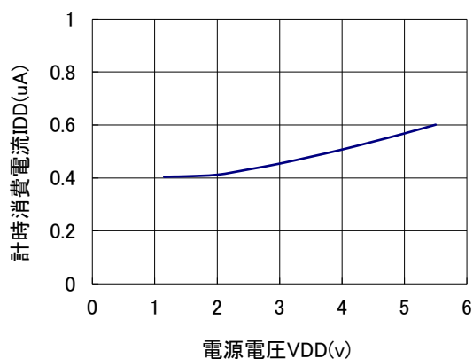
計時消費電流 vs 電源電圧特性(32K クロック非出力時) (出力=Open, T_{opt}=25^{\circ}\text{C} )
