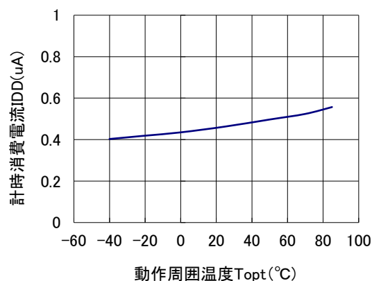
計時消費電流 vs 周囲温度特性(32K クロック非出力時) (出力=Open, VDD=3V)
