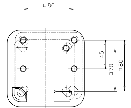
取付部詳細図 (S=1:3)
