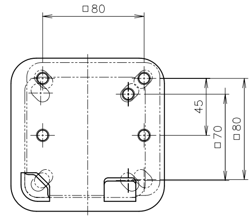
取付部詳細図 (S=1:3)
