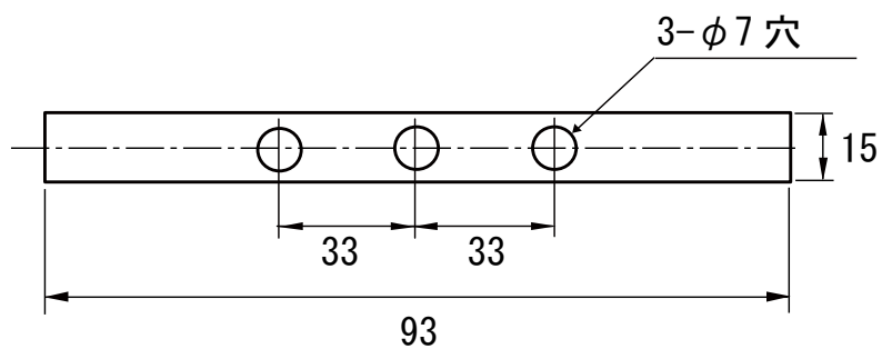
取付穴寸法
