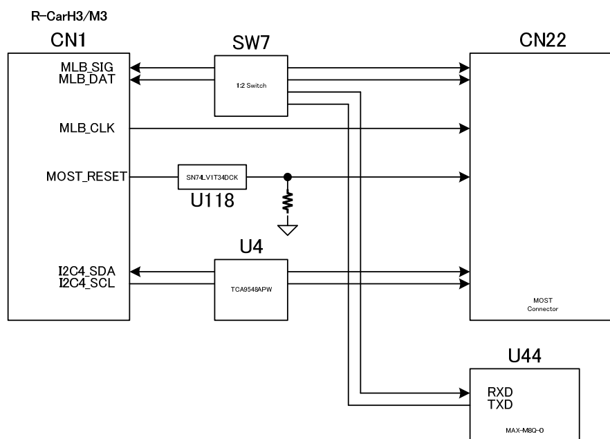
図 4-17 MOST I/F
