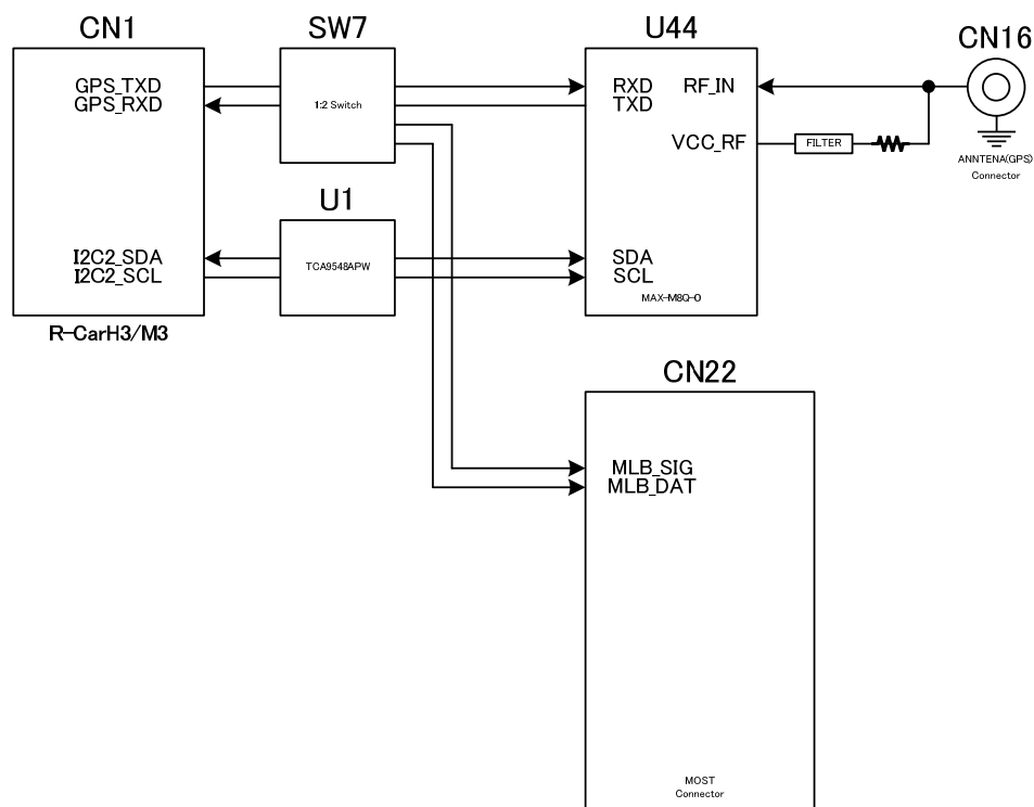
図 4-18 GPS I/F
