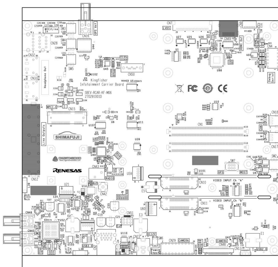
图 9a 基板表面图
