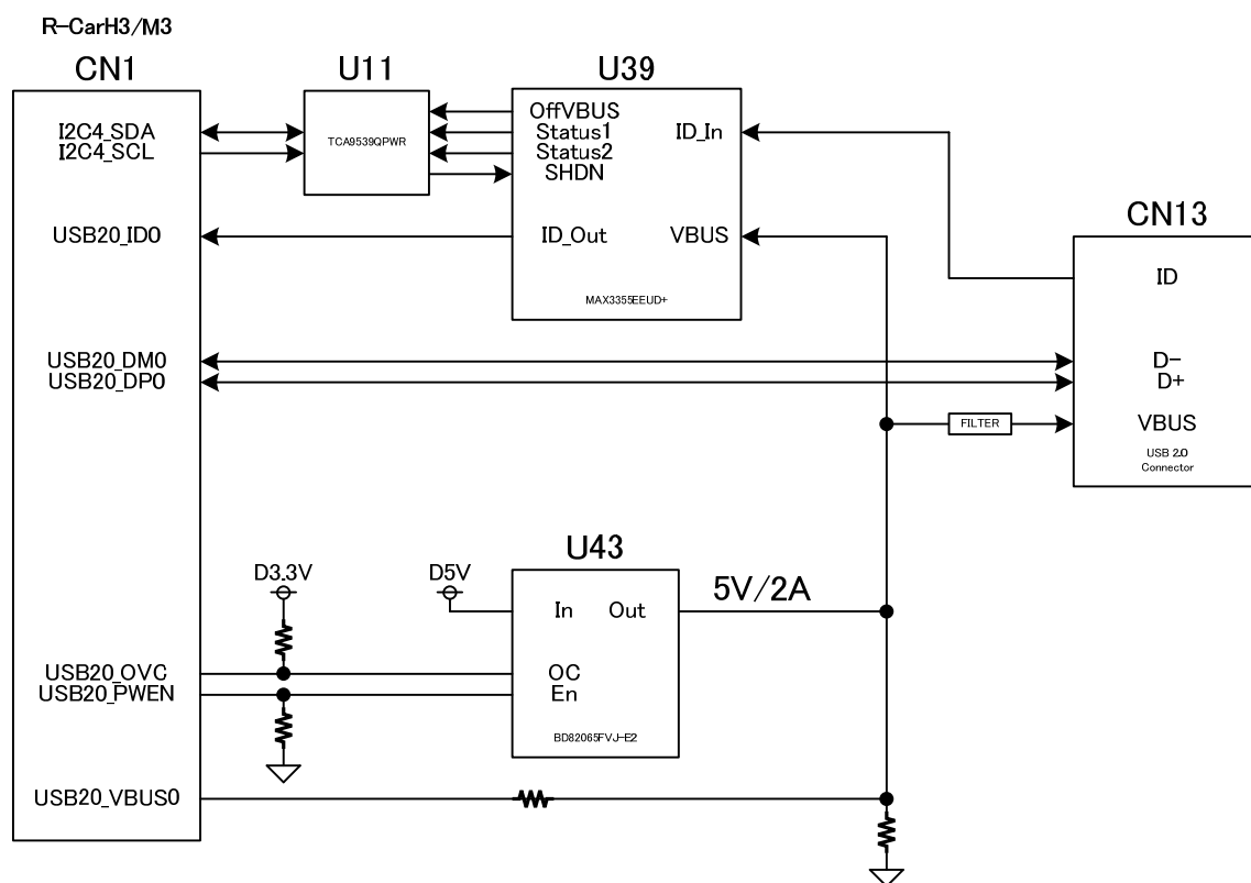
图 4-5 USB 2.0 I/F
