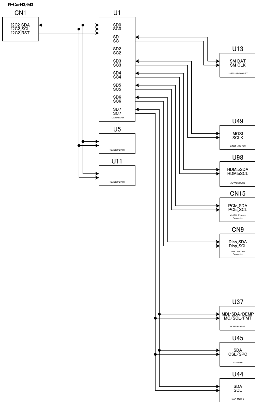
図 4-21a I2C I/F
